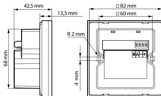
Puszka montażowa do montażu natynkowego
