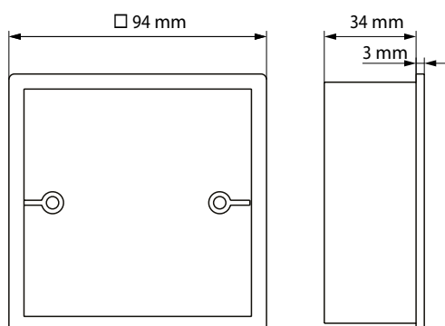
Puszka montażowa do montażu podtynkowego
