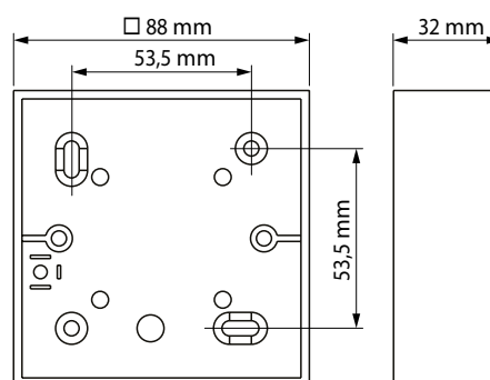
Puszka montażowa do montażu natynkowego
