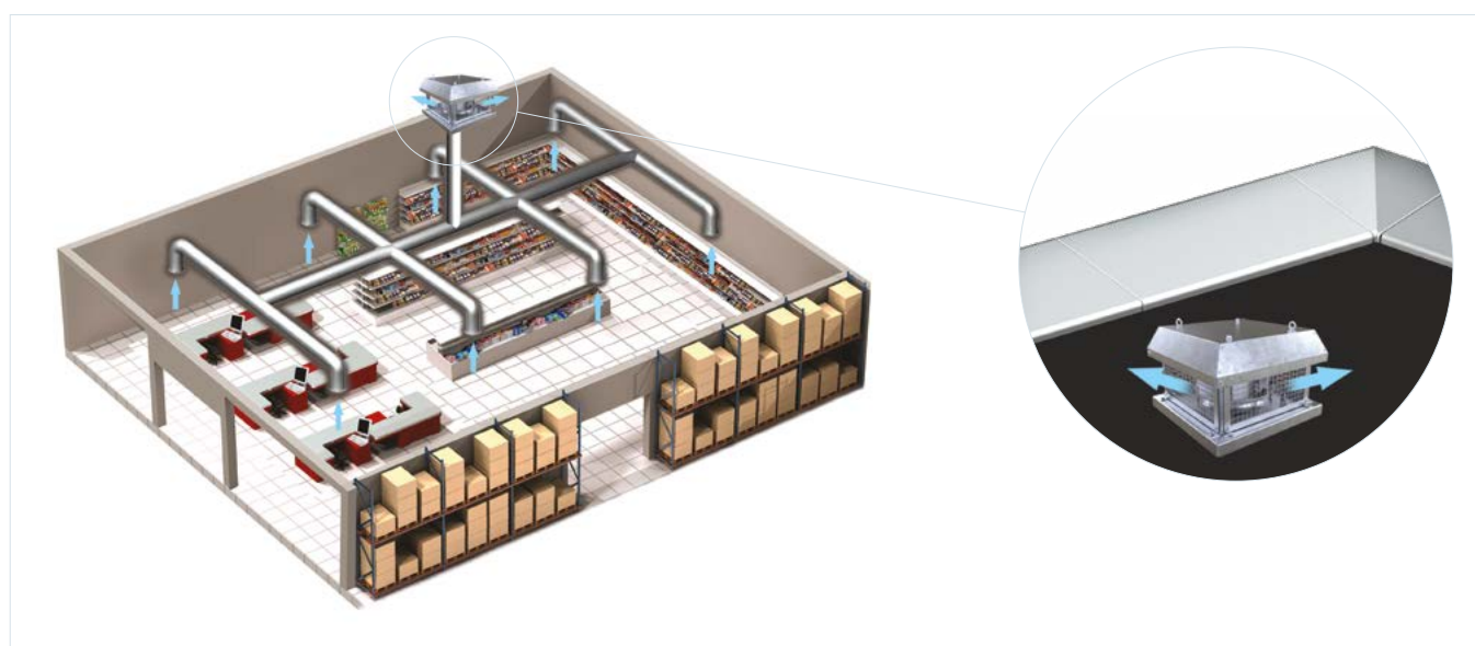
Przykład systemu wentylacyjnego z użyciem wentylatora VKHz EC
