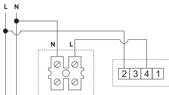
Wentylator pracuje od momentu osiągnięcia progu temperatury podanego w termostacie
