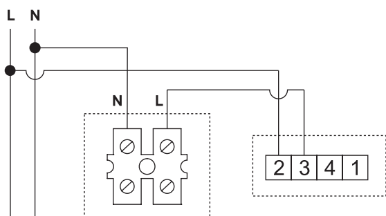
Wentylator pracuje do momentu osiągnięcia progu temperatury podanego w termostacie
