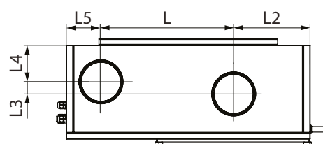
Widok B (strona podłączenia do pomieszczenia)
