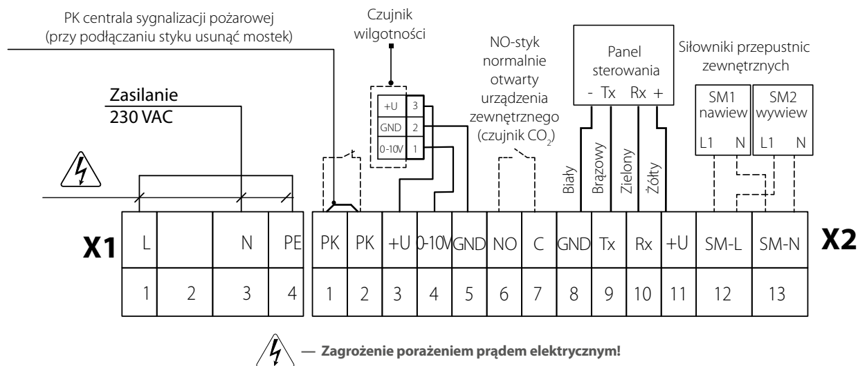
Schemat połączeń zewnętrznych central VUT 160/250/350 PB EC A21
