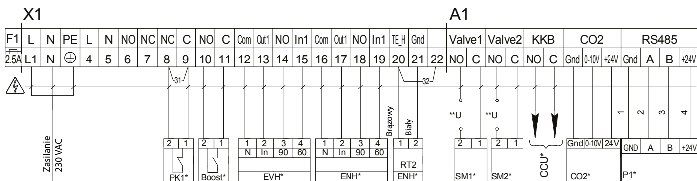
Schemat połączeń zewnętrznych central VUT 160/250/350 PB EC A21
