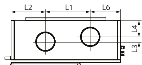
Widok A (strona podłączenia na zewnątrz)
